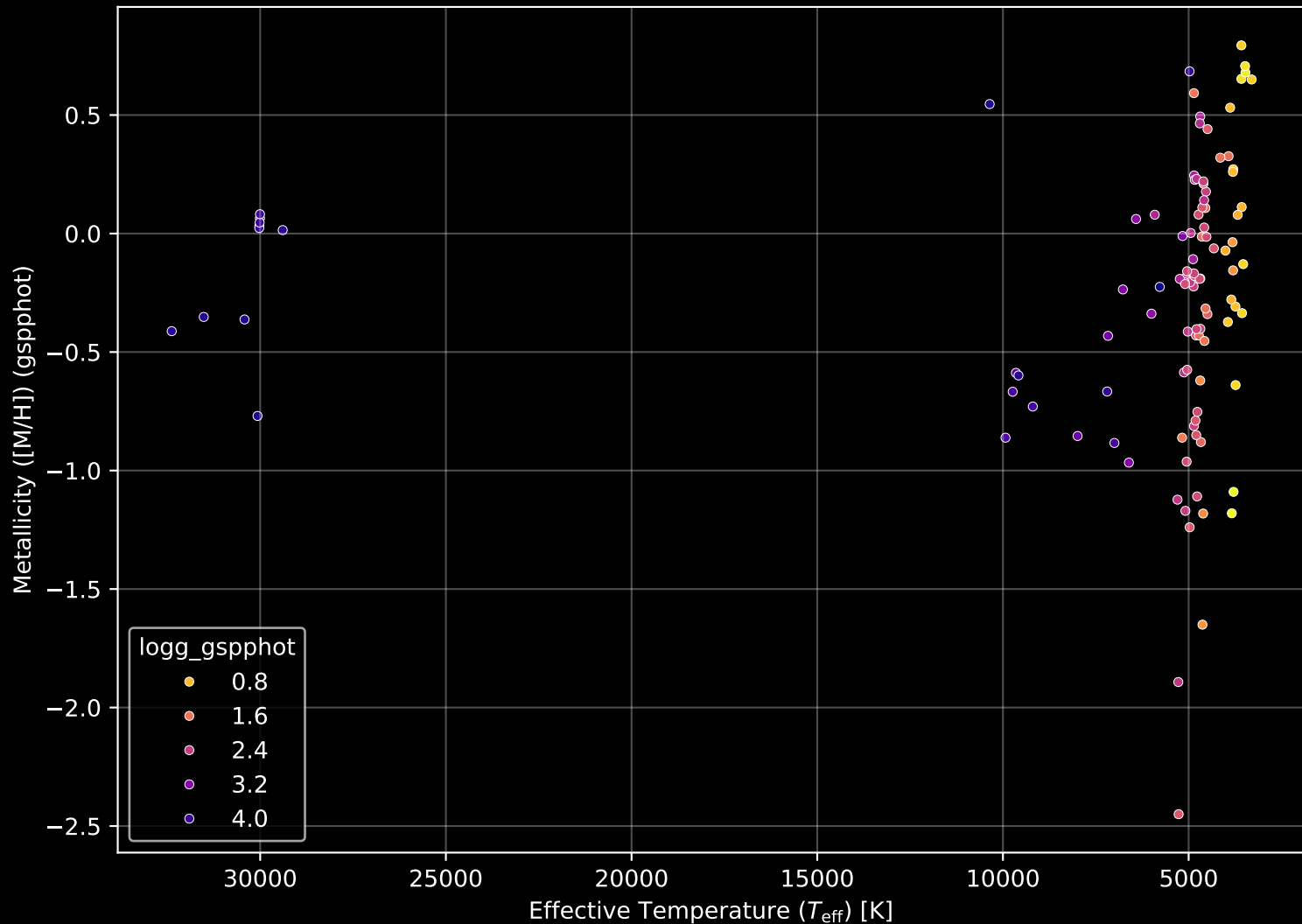
APOGEE DR17 Field: [005+03] Stellar Population Parameters (n= 108)
